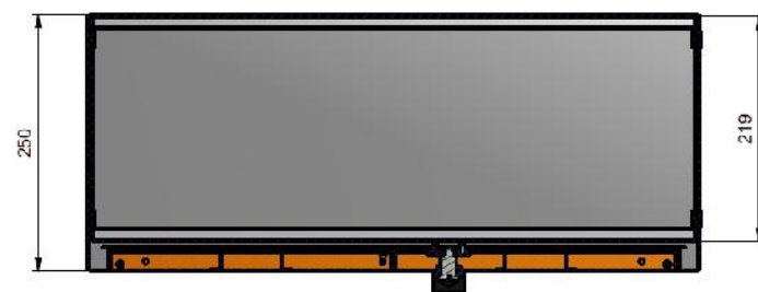
B-B ( 1 : 5 )
