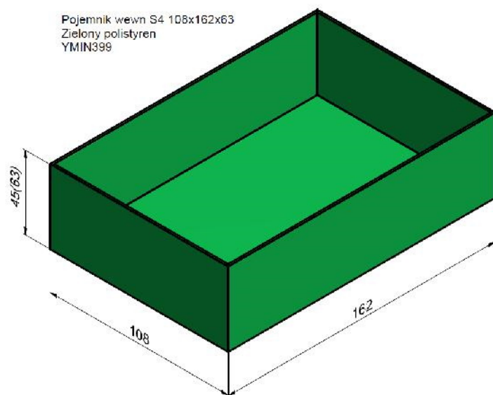
Pojemnik wewn S4 108x162x45 Zielony polistyren YMIN398
