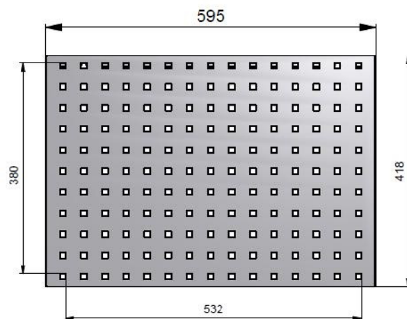
wyk.B Ścianka perforowana w. - XSWW 2200262701
