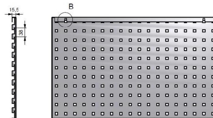
A-A (0,17 : 1)
