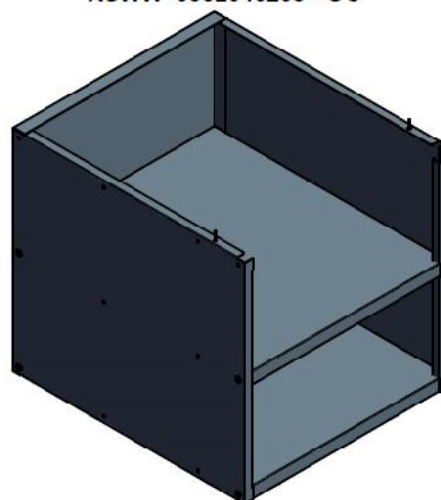
wyk. F (tył, 2 półki)
