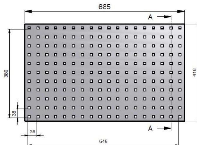
wyk.A Ścianka perforowana s. - XSWW 2200272701
