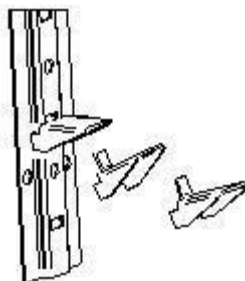
Rys. 2. Montaż zaczepu półki.
