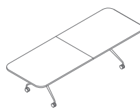
PCZ03 2800 / 1000 / 740** 94 kg
