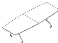
PCB03 2800 / 1000 / 740** 94 kg
