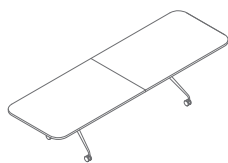
PCZ05 3200 / 1000 / 740** 101 kg
