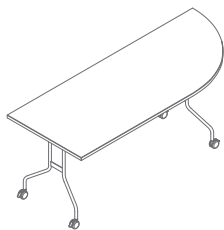
PFT05 2000 / 800 / 740 42.75 kg
